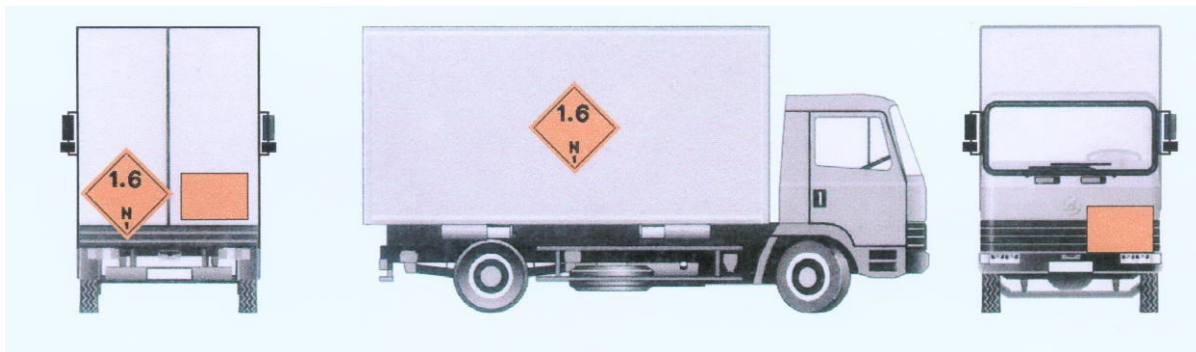
Obrázok č. 5 : Označenie vozidla pri preprave výbušných látok
